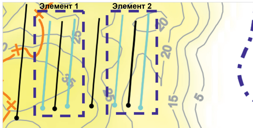
Рис. 5. Участок ОПР по полимерному заводнению Fig. 5. Polymer flooding pilot area
