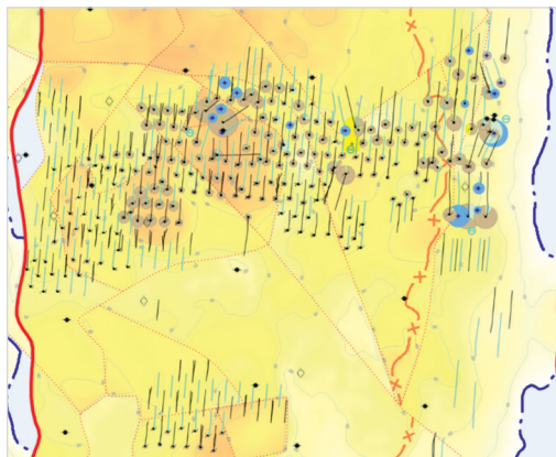
Рис. 4. Карта накопленных отборов по состоянию на 01.08.2020 г. Fig. 4. Bubble map as of 01.08.2020
