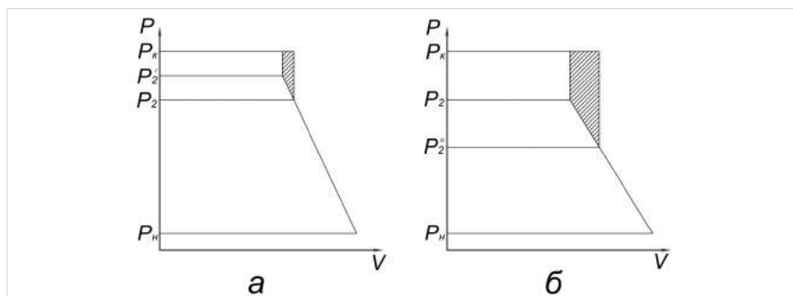
Рис. 1 — Теоретические индикаторные диаграммы винтового маслозаполненного компрессора: а — без конденсации газа в рабочих ячейках; б — при конденсации газа в рабочих ячейках.
