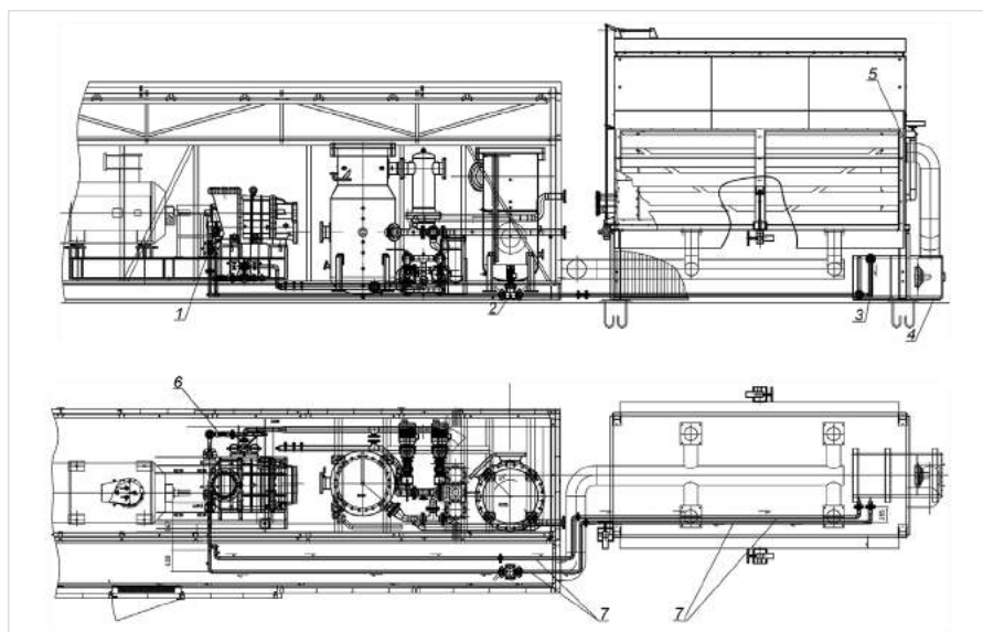
Рис. 2 — Дополнительно установленные элементы системы теплообмена: 1 — жидкостной теплообменник; 2 — насос жидкости; 3 — жидкостной радиатор; 4 — вентилятор; 5 — воздуховод; 6 — мембранный расширительный бак для жидкости; 7 — соединительные трубопроводы
