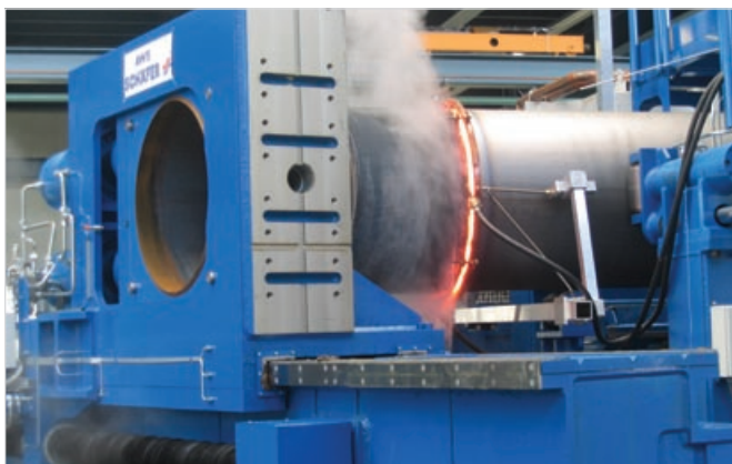
Рис.2 – Стан SRBMI 800 для изготовления гнутых отводов
