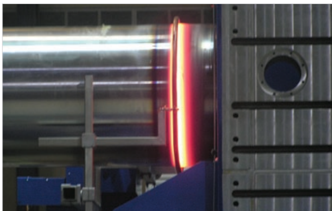
Рис.4 – Сталь 15Х1М1Ф
