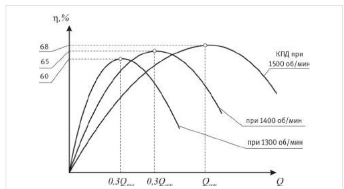
Рис. 4 — Зависимости КПД насоса от его производительности при различных скоростях вращения рабочего колеса
