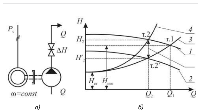
Рис. 1 — Регулирование производительности насосного агрегата с помощью задвижки: а) Функциональная схема; б) Характеристики насоса и магистрали
