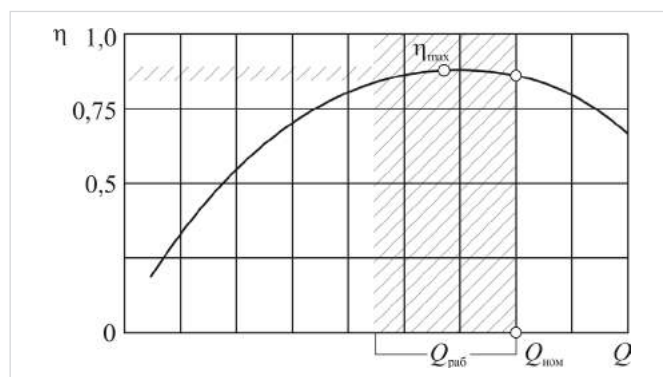
Рис. 2 — Зависимость КПД насоса от его производительности
