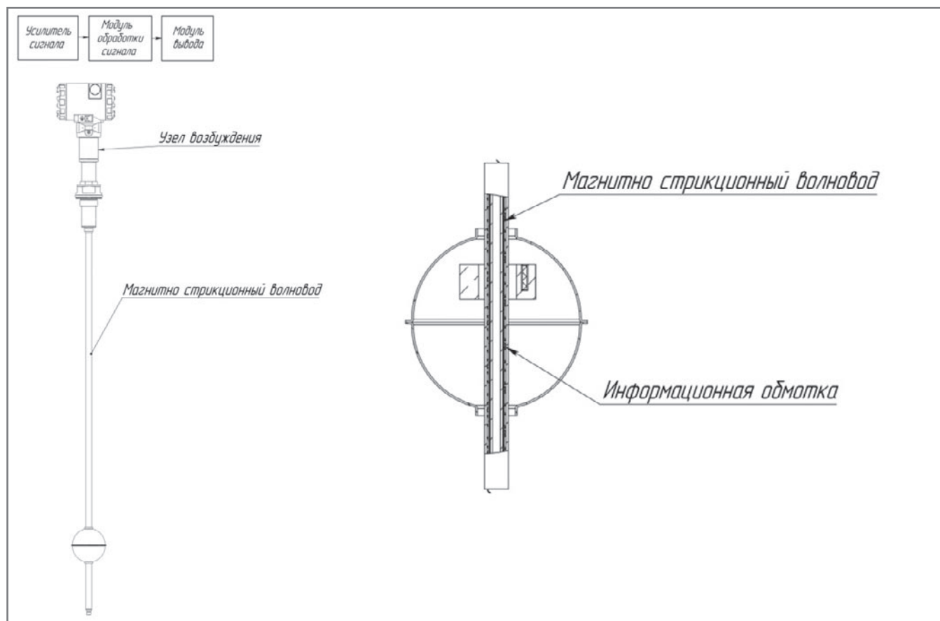
Рис. 1. Магнитострикционный преобразователь производства ООО «Первая Приборная фабрика»
