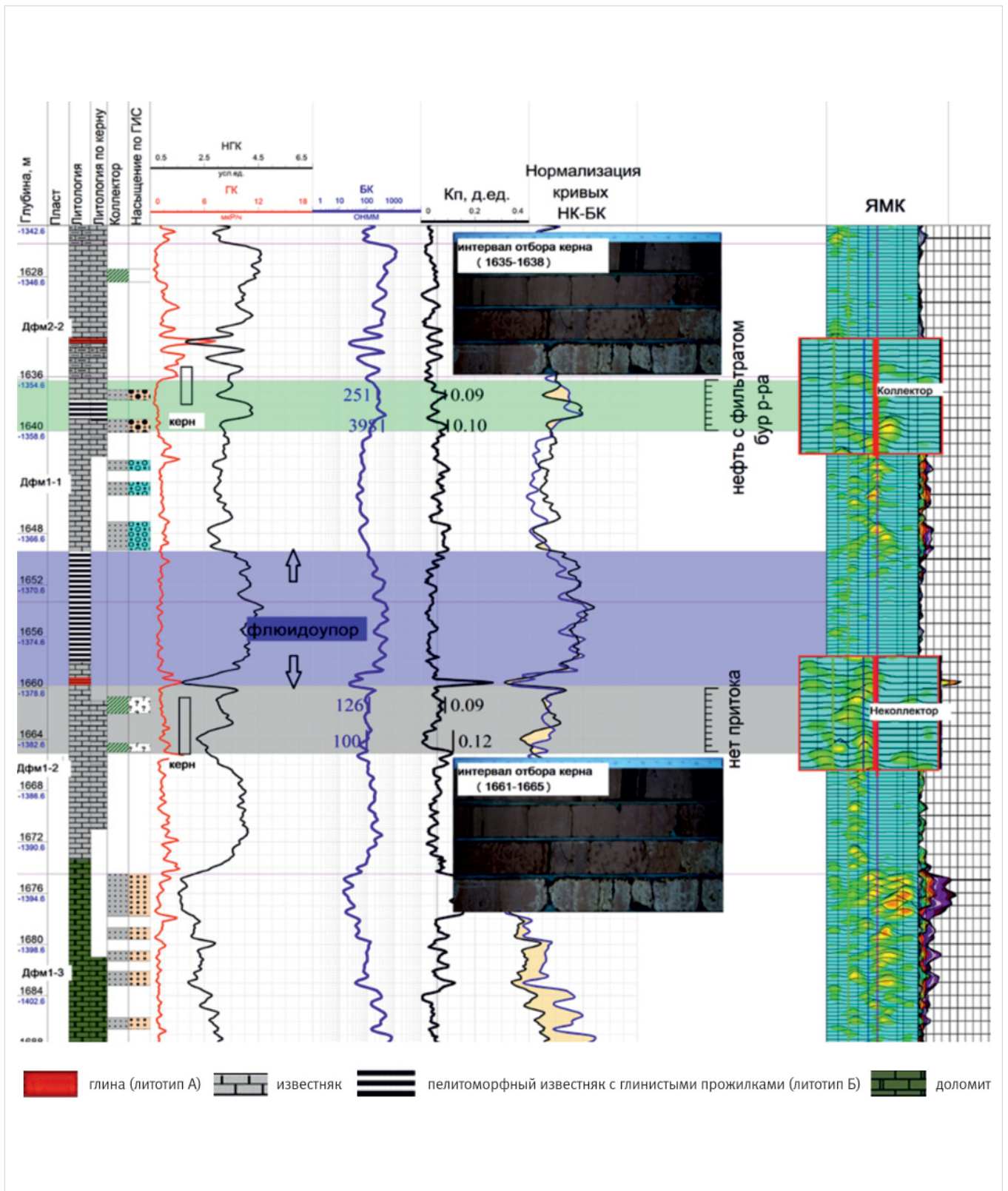
Рис. 7. Пример использования ядерно-магнитного метода для снижения неоднозначности выделения коллектора и насыщения Fig. 7. An example of the use of nuclear magnetic logging as a method to reduce the ambiguity of reservoir identification and saturation
