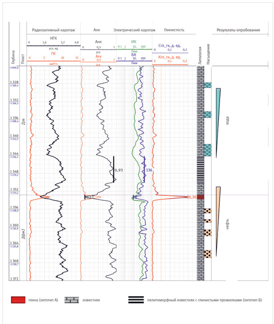
Рис. 3. Выделение флюидопоров по методам ГИС на примере скважины 3** Fig. 3. Selection of the seal rock on the example of well 3**
