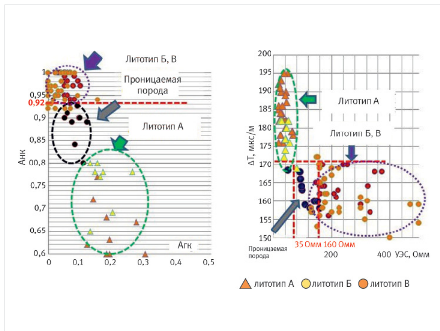
Рис. 6. Распределения геофизических параметров пород, слагающих флюидоупор в разрезе верхнедевонской карбонатной толщи Fig. 6. Distributions of geophysical parameters of rocks composing the fluid seal in the section of the Upper Devonian carbonate strata
