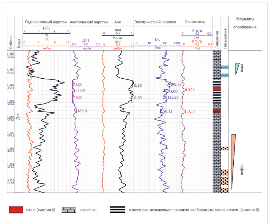
Рис. 4. Выделение флюидопоров по методам ГИС на примере скважины 4** Fig. 4. Selection of the seal rock on the example of well 4**
