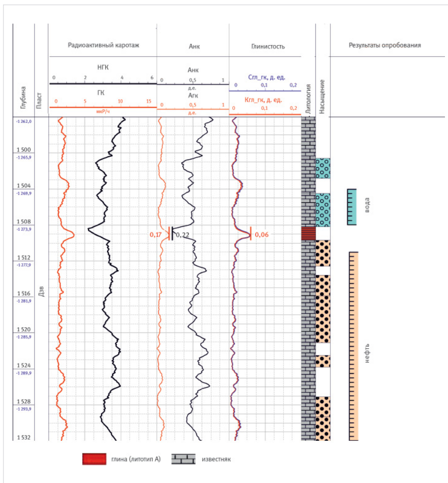
Рис. 2. Выделение флюидоупора на примере скважины 2** Fig. 2. Selection of the seal rock on the example of well 2**
