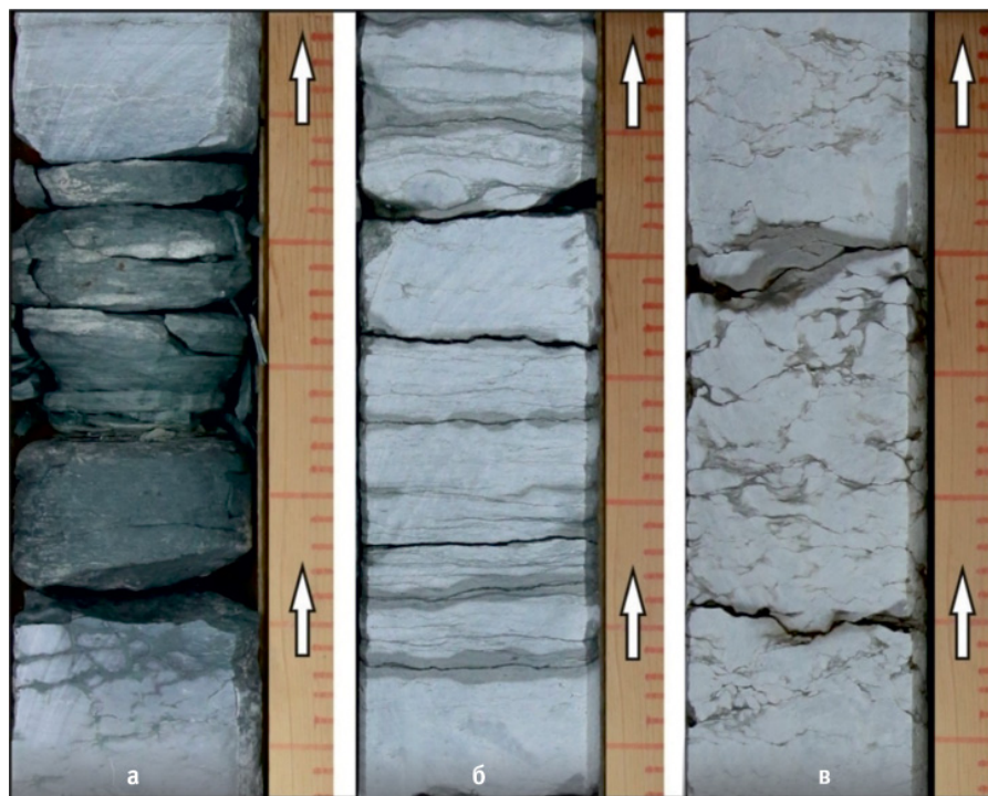
Рис. 1. Литологические типы флюидоупоров фаменского яруса: а — глины известковые, б — известняки пелитоморфные с глинистыми прожилками, в — известняки желваковые с глинисто-карбонатным заполнителем. Цена деления линейки — 1 см, стрелки направлены от подошвы к кровле
