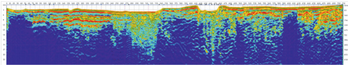
Рис. 2. Георадарный разрез по оси скважины Fig. 2. Georadar section along the axis of the well
