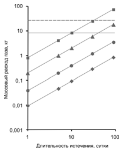
Рис. 3. График зависимости массы газа вытекающего с конца кабеля в невзрывоопасной зоне от времени при давлении во взрывоопасной зоне и длине кабеля
