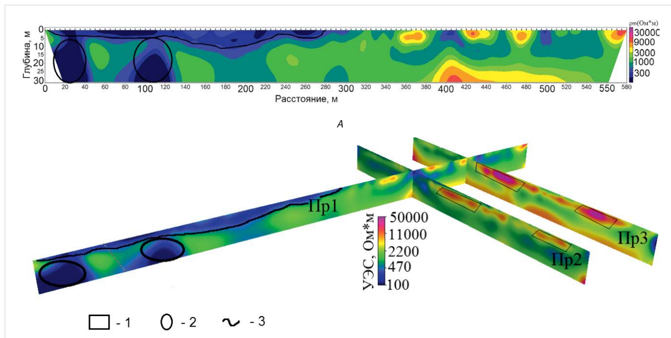
Рис. 5: А — Геоэлектрический разрез по профилю №1, Б — Трехмерная визуализация геоэлектрических разрезов. 1 — линзы подземных льдов, 2 — аномальная область от металлических коммуникаций, 3 — кровля многолетнемерзлых грунтов Fig. 5: A — Geoelectric section on profile № 1, B — three-Dimensional visualization of geoelectric sections. 1 — lenses of underground ice, 2 — anomalous area from metal communications, 3 — the roof of permafrost
