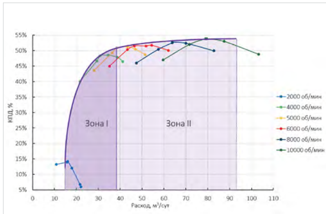
Рис. 3 — КПД насосной установки в диапазоне частот 2000–10000 об/мин Fig. 3 — ESP efficiency in speed shaft range 2000–10000 rpm
