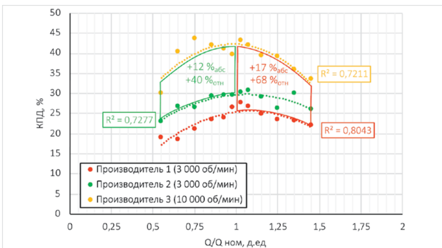
Рис. 2 — КПД-характеристика УЭЦН различных производителей с номинальной подачей менее 100 м³/сут
