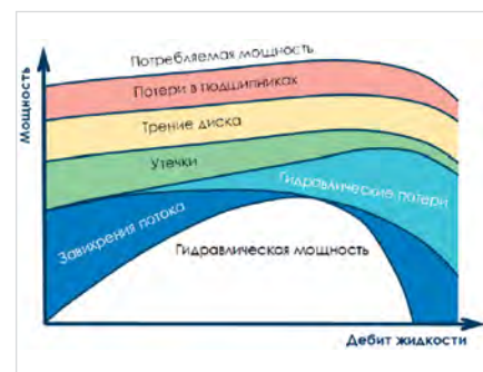
Рис. 1 — «Качественная картина» потерь энергии в ЭЦН Fig. 1 — Energy losses of ESP
