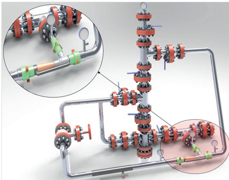
Рис. 1. УСУ в устье обвязке скважины
