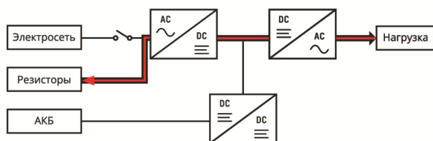
Рассеивание энергии на резисторах
