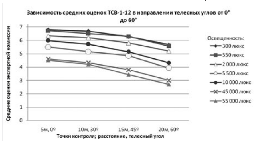
Рис. 3 — Зависимость оценок качества восприятия текстовой информации с табло TCB-1-12 на разных точках контроля в условиях разной освещенности
