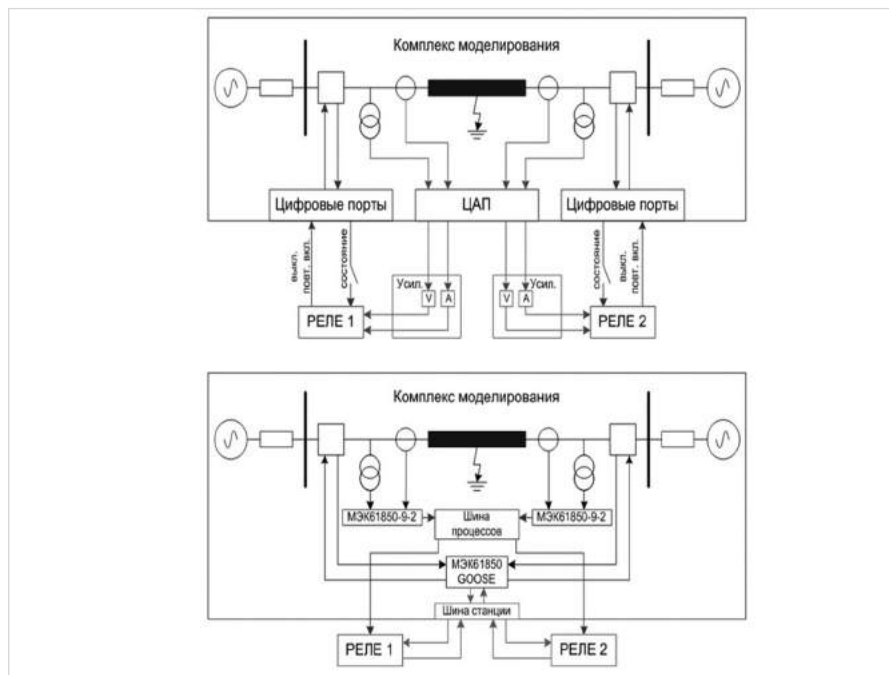
Рис. 1 — Примеры подключения внешнего оборудования к КМРВ
